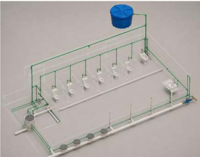
Projeto Hidrossanitário - Banheiros
