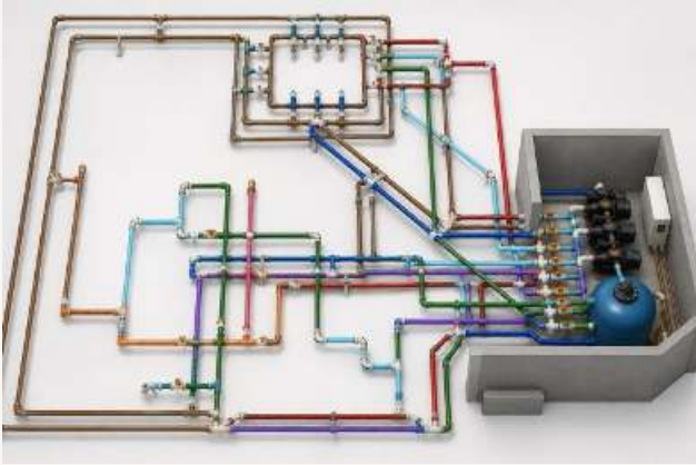
Piscina – hidrossanitário
