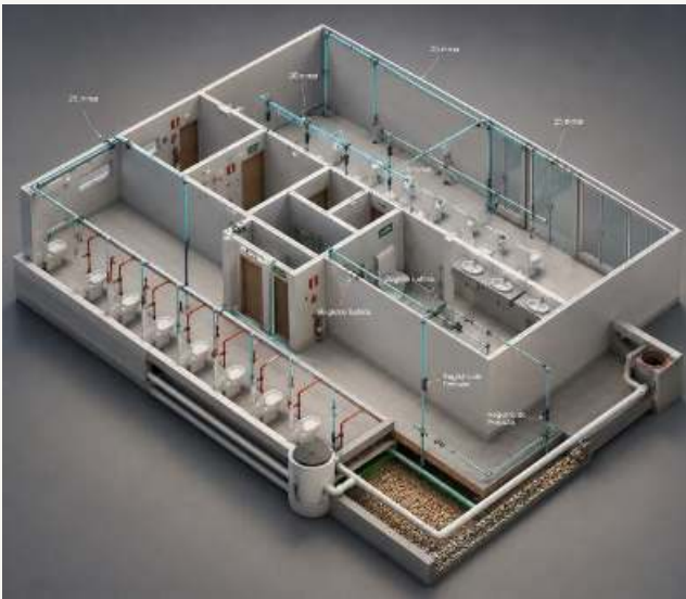
Projeto Hidrossanitário - Banheiros
