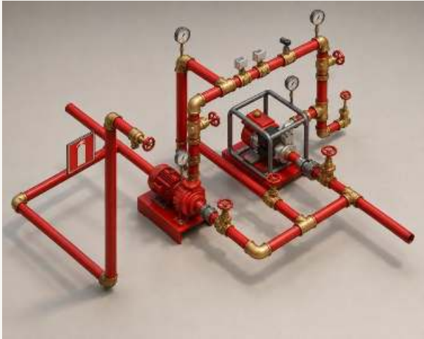
Bombas de Incêndios - Isométrico
