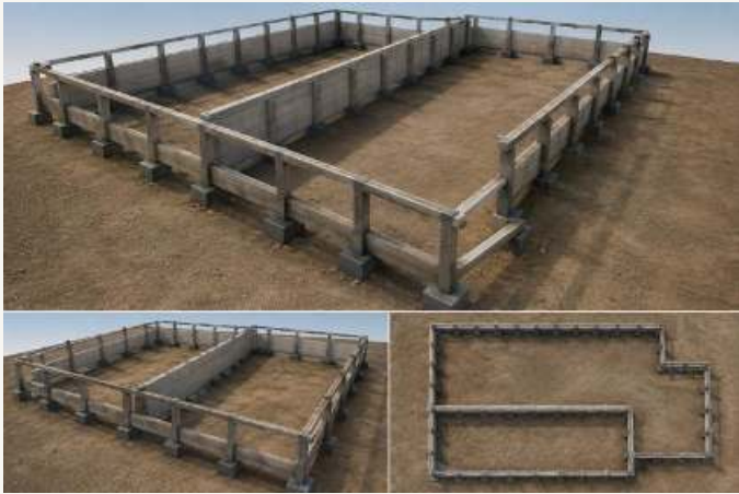
Contenção
