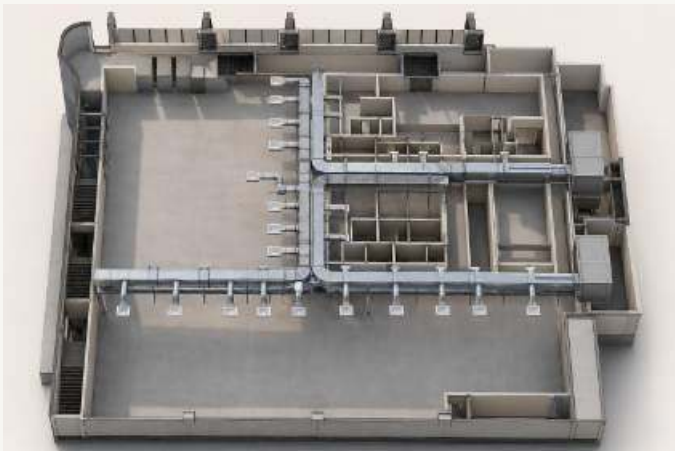
Dutos de Refrigeração
